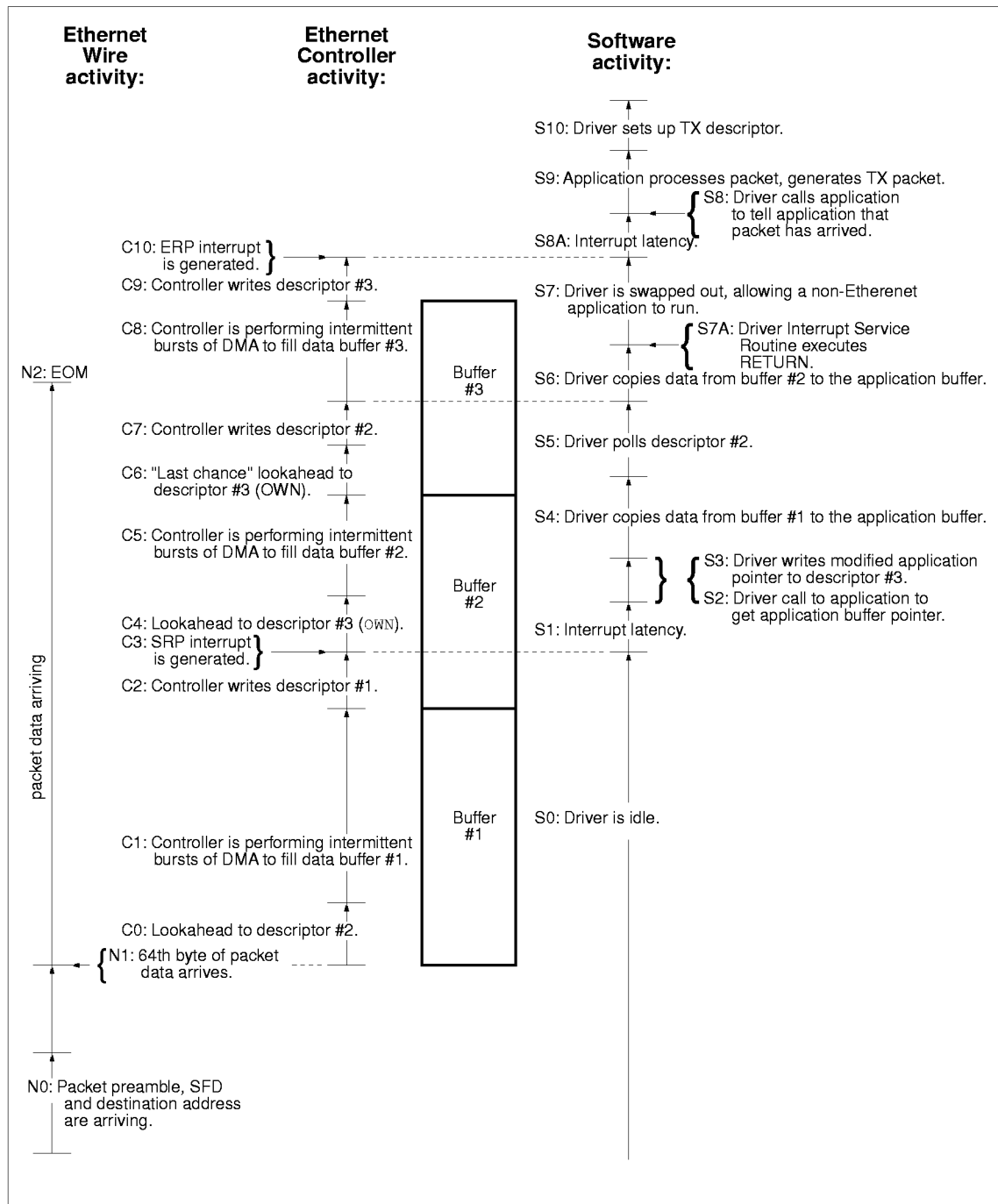
Figure D1. LAPP Timeline
