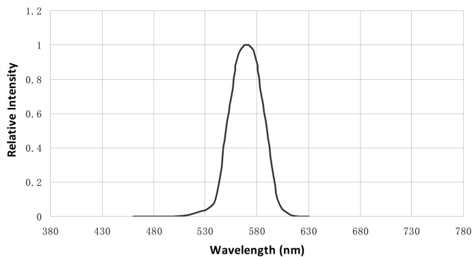
光谱分布特性曲线
