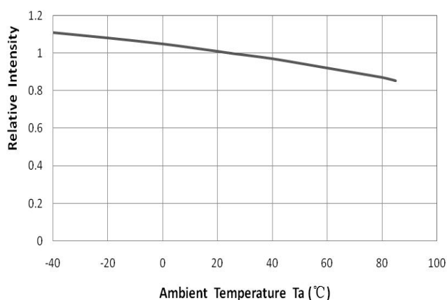
相对光强与环境温度特性曲线
