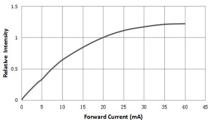
相对光强与电流特性曲线
