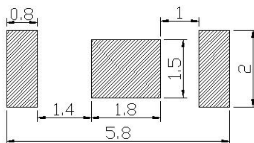
焊盘建议图
