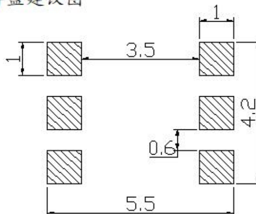
焊盘建议图
