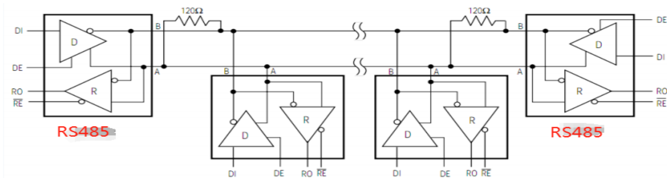
图 11 典型的 RS485 半双工通讯网络
