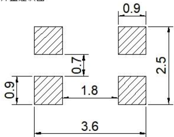
焊盘建议图
