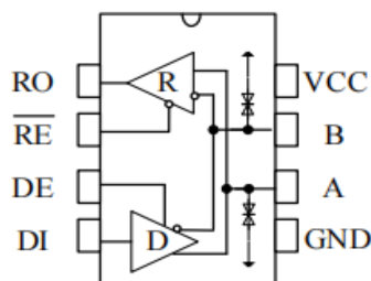
图 1 引脚分布图
