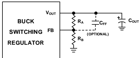
图 26. 反馈电阻网络
