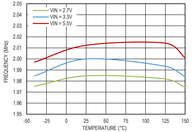
图 13. 频率和温度的关系，RT 接高
