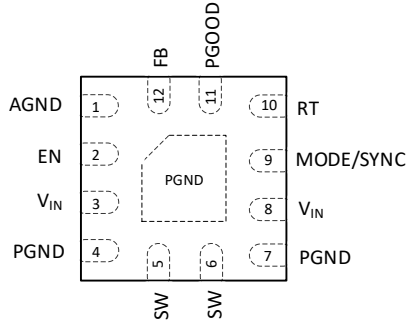
12 引脚 LQFN (2mm x 2mm)
