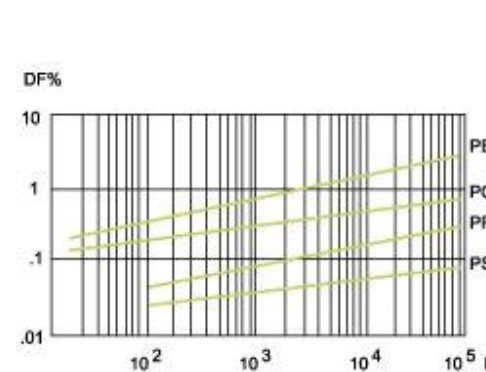
损耗角正切与频率的关系 Dissipation Factor vs. Frequency
