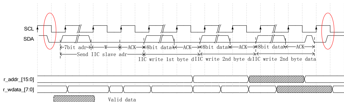
图一 I2C 写寄存器时序
