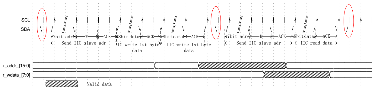
图二 I2C 读寄存器时序
