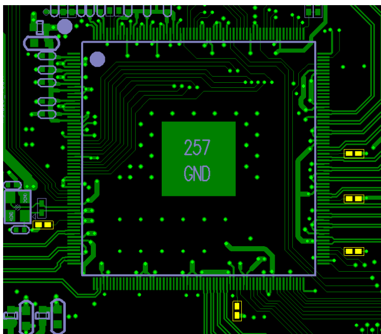
图十一 REXT 电阻 PCB 绘制示意图
