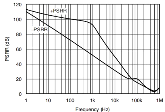
Figure 4. 电源抑制比与频率间的关系
