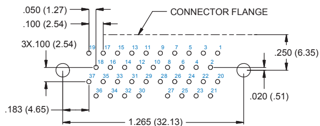
37 SOCKET
