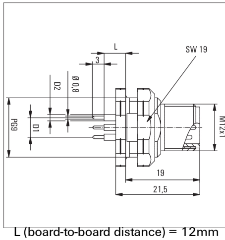
Front panel section D1 = 5,5 mm D2 = 1,4 mm
