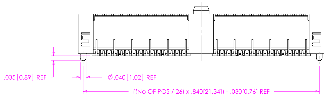
FIG. 1 QFSS-052-01-X-D-A SHOWN
