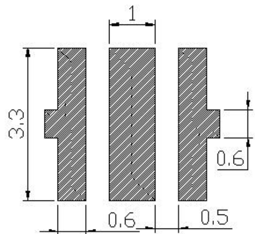
焊盘建议图
