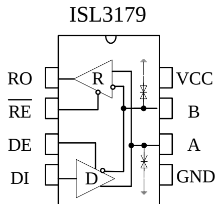
图 1 引脚分布图
