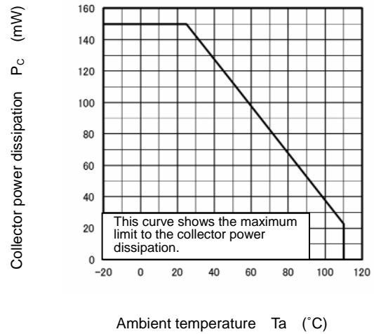
P_C - T_a
