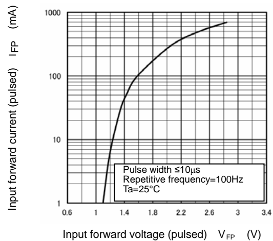
I_{FP} - V_{FP}
