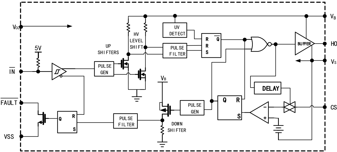
图 10-1 功能框图
