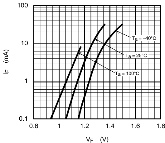
Fig. 12.3 I_F - V_F
