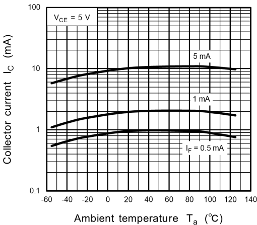
Fig. 11.13 I_C - T_a
