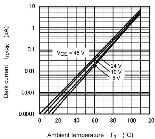
Fig. 11.11 I_{DARK} - T_a
