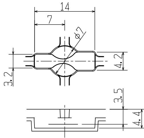
Detail A (2:1) 詳細 A (2:1)
