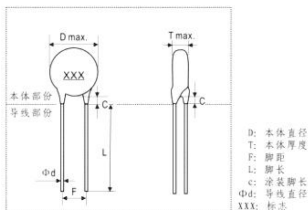
外形尺寸图
