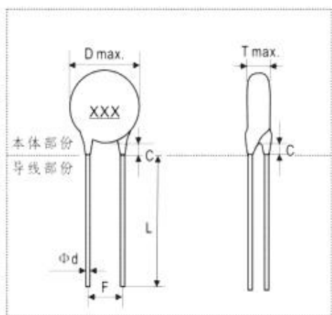
外形尺寸图
