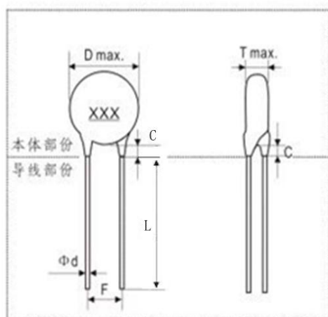
外形尺寸图
