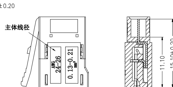
A-A SECTION
