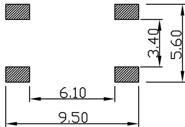
PCB. 焊接图
