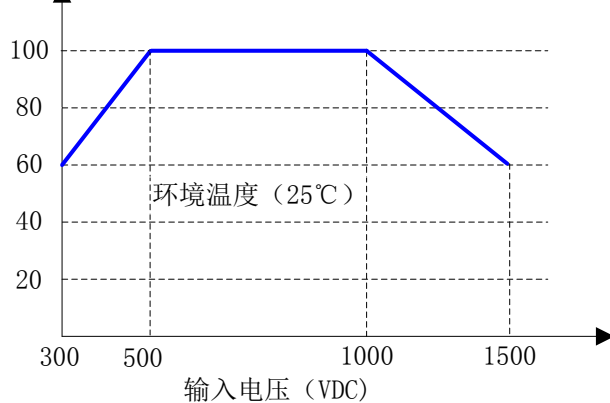
负载随输入电压降额曲线图
