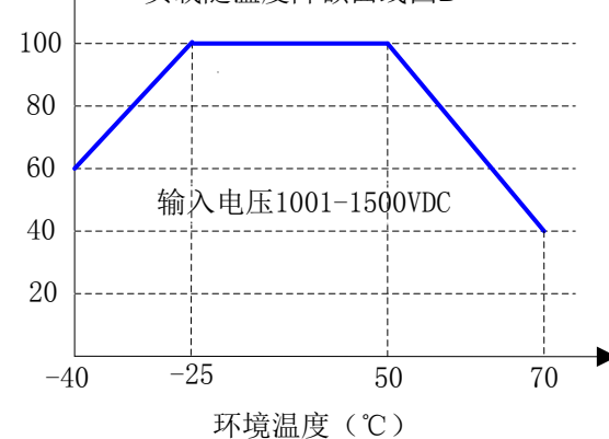
负载随温度降额曲线图B
