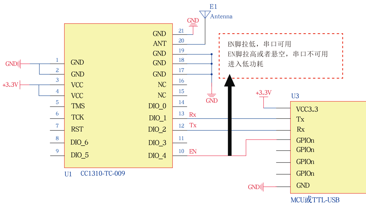
图 2 普通透传模块式
