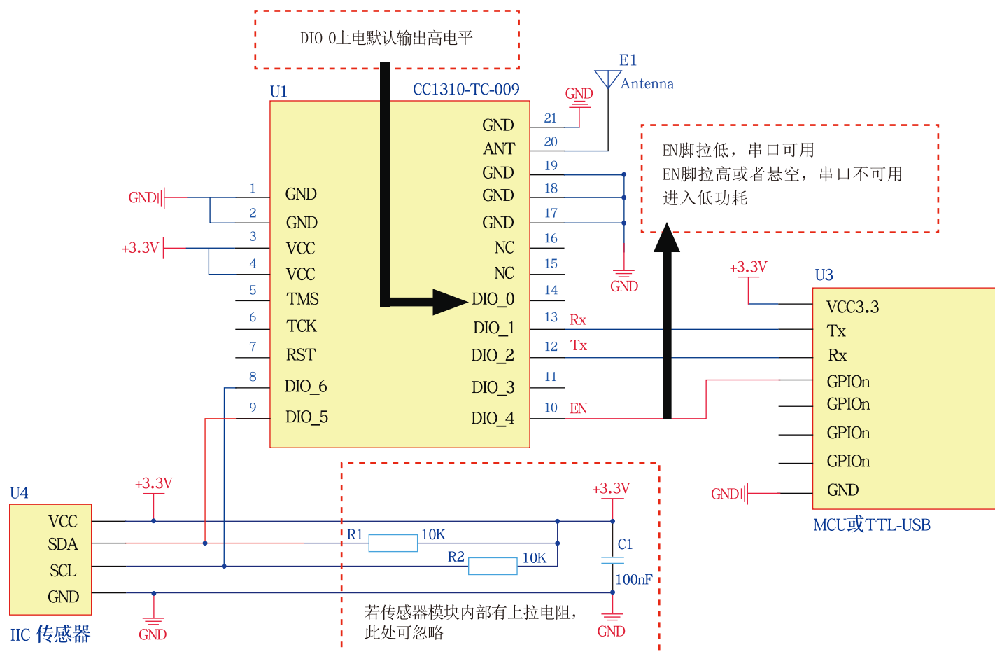
图 4 I2C传感器模式
