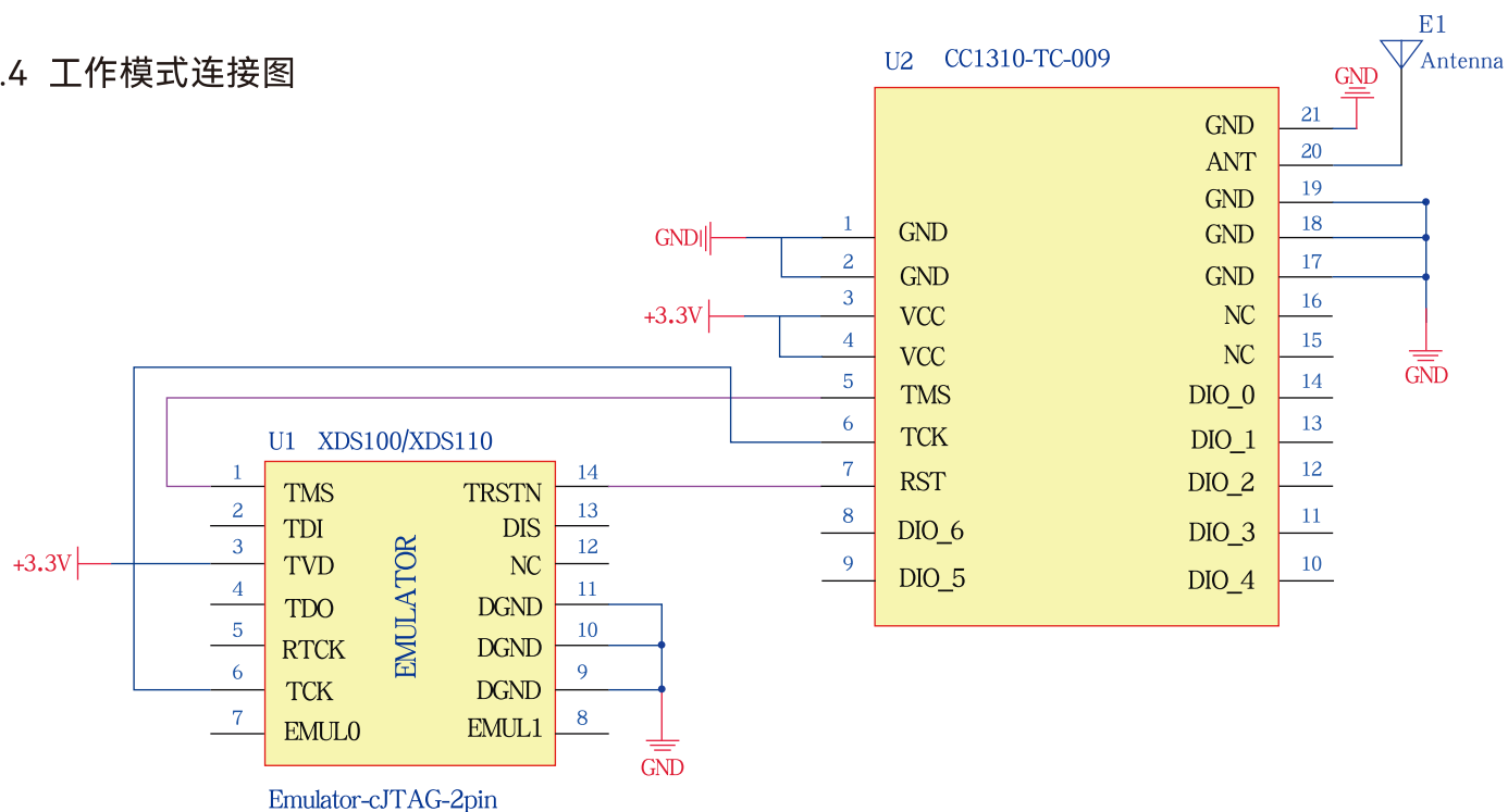
图 1 二次开发接线图
