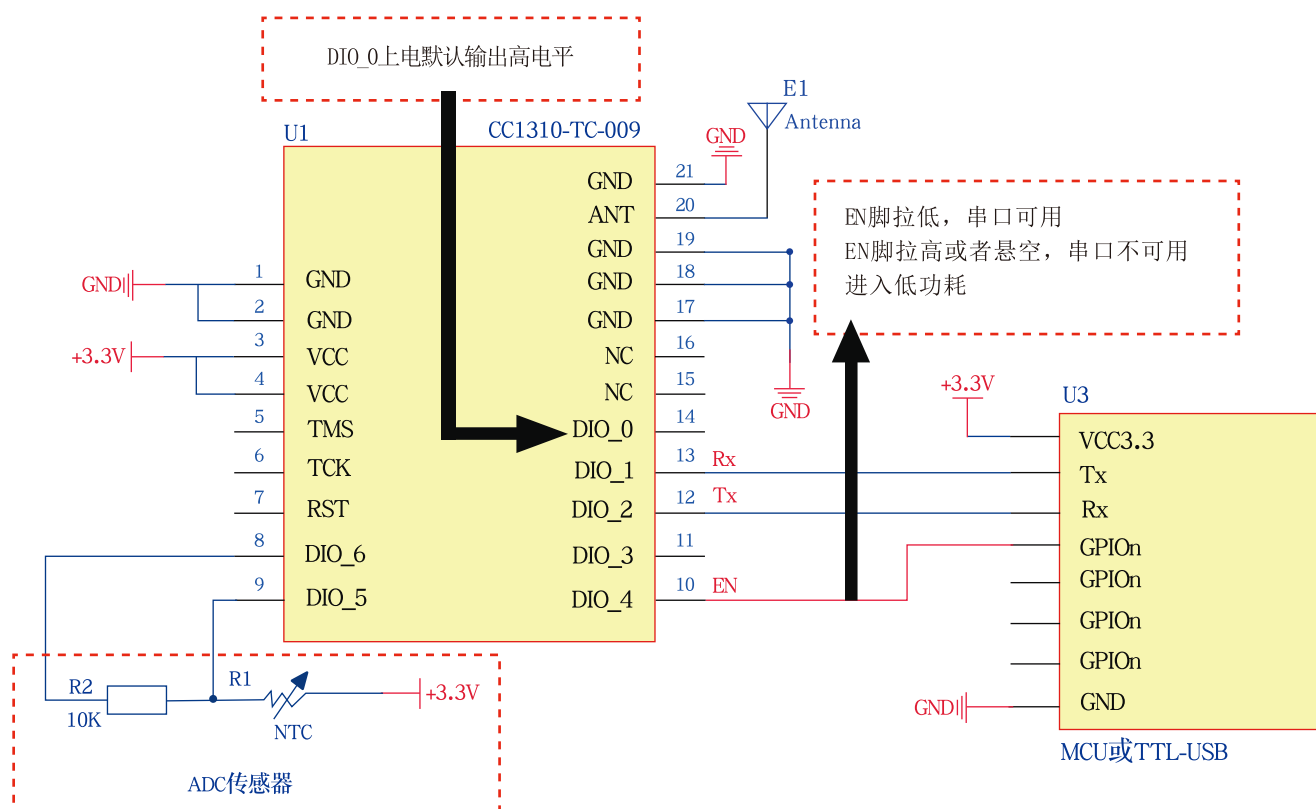
图 3 ADC传感器模式
