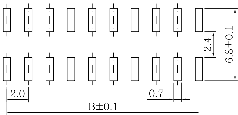
P.C.B Layout
