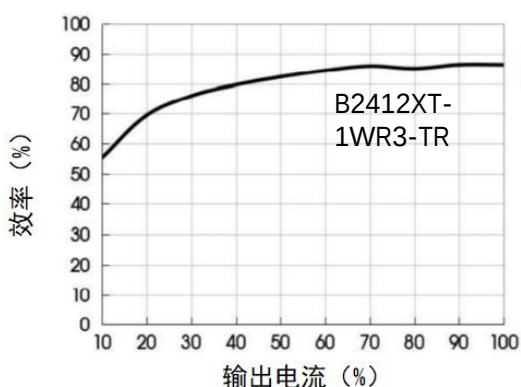
效率 VS 输出负载曲线图 (Vin=24V)
