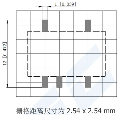
PCB 印刷版图
