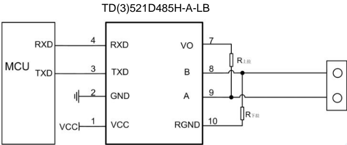
图1.典型应用电路
