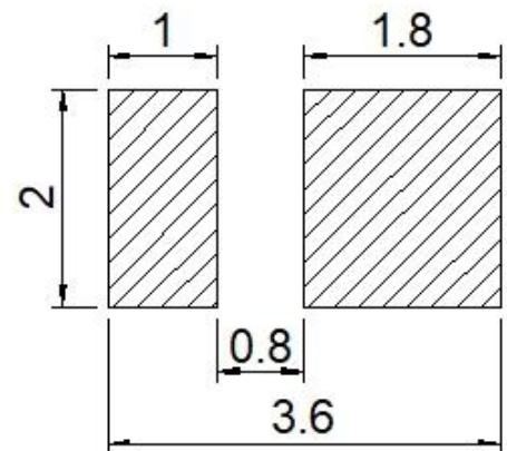
焊盘建议图
