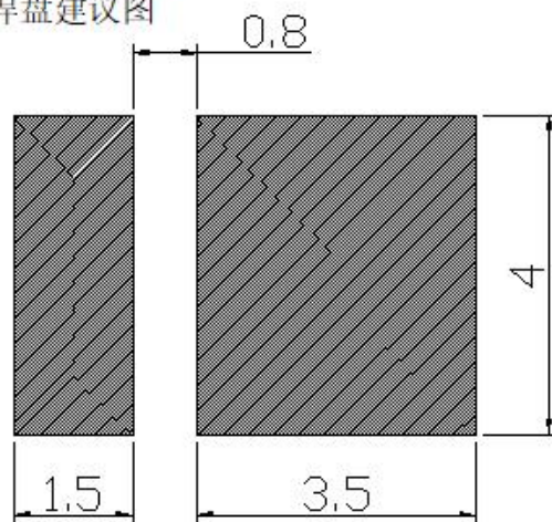
焊盘建议图
