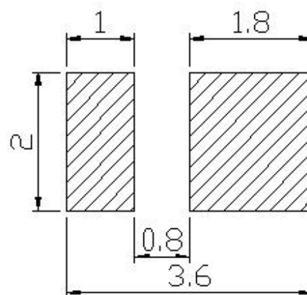
焊盘建议图
