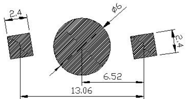
焊盘建议图
