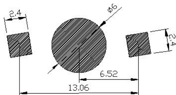
焊盘建议图
