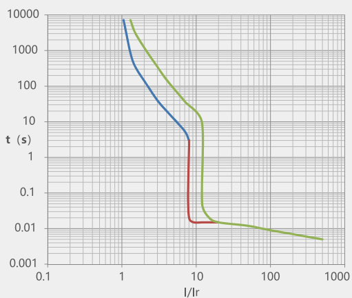
图 33 NM1-800 配电保护
