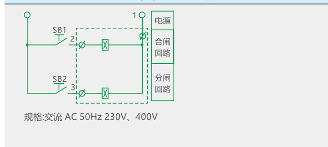
NM1-63、125、250 电动操作机构 (AC) 分、合闸原理图
