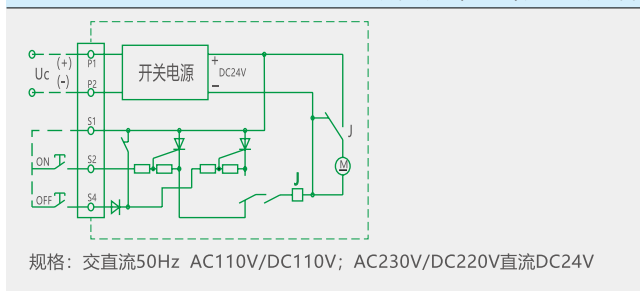
NM1-63、125、250、400、630、800、1250 电动操作机构 (AC/DC) 分、合闸原理图
