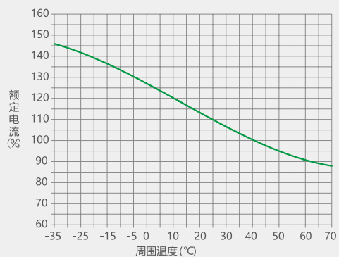
图 34 NM1-800 温度补偿曲线
