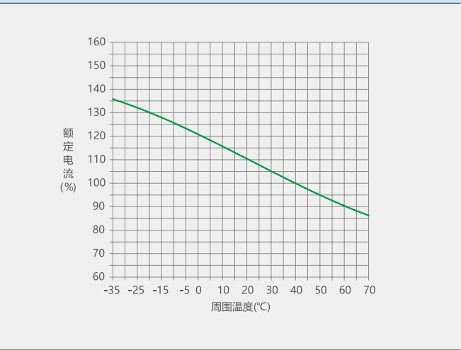
图 2 NM1-63 10A-25A 温度补偿曲线
