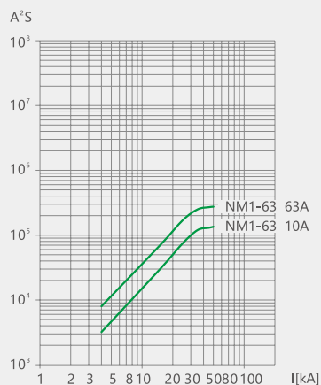
图 40 NM1-63 允通曲线
