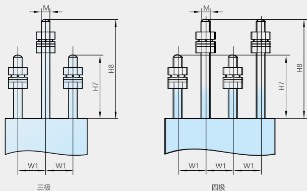
NM1-400、630、800外形及安装尺寸(板后接线)(见表10)
