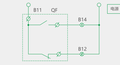
报警触头接线图
