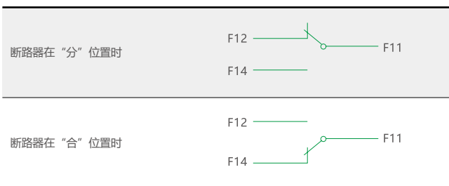
辅助触头接线图
