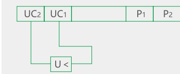
欠电压脱扣器接线图
