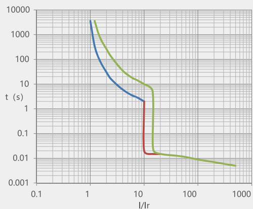
图 11 NM1-125 16A 电动机保护
