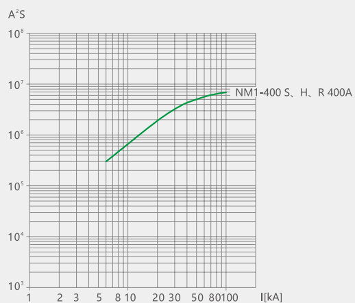
图 43 NM1-400 允通曲线
