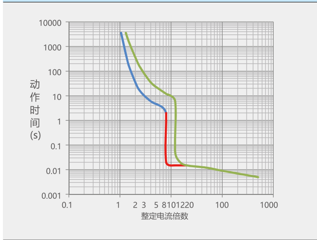
图 1 NM1-63 10A~25A 配电保护
