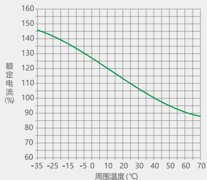
图 36 NM1-800 温度补偿曲线
