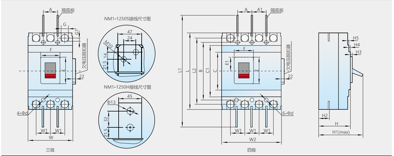
NM1-400、630、800、1250外形及安装尺寸(板前接线)(见表9)
