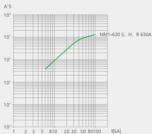
图 44 NM1-630 允通曲线
