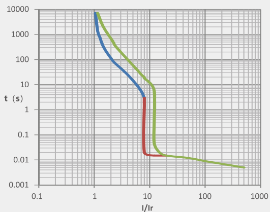
图 31 NM1-630 配电保护
