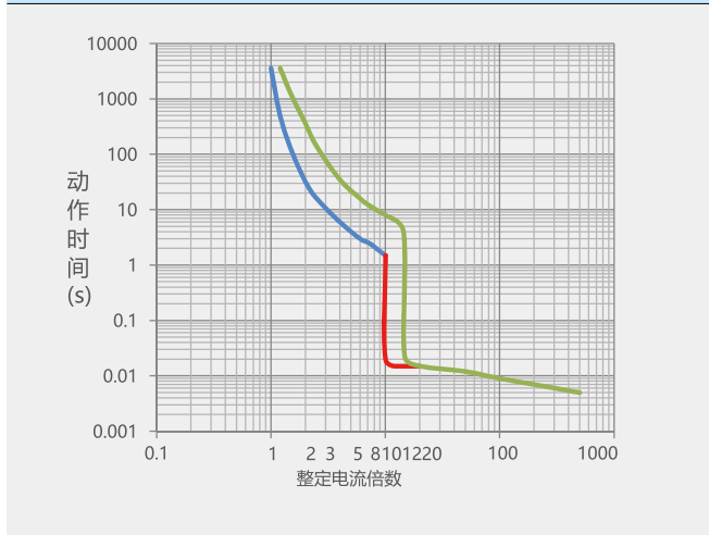
图 3 NM1-63 10A~25A 电动机保护
