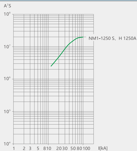
图 46 NM1-1250 允通曲线
