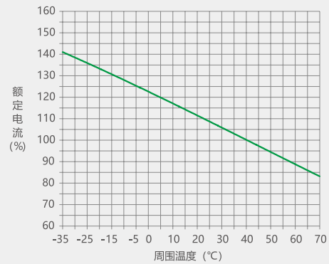
图 26 NM1-400 温度补偿曲线
