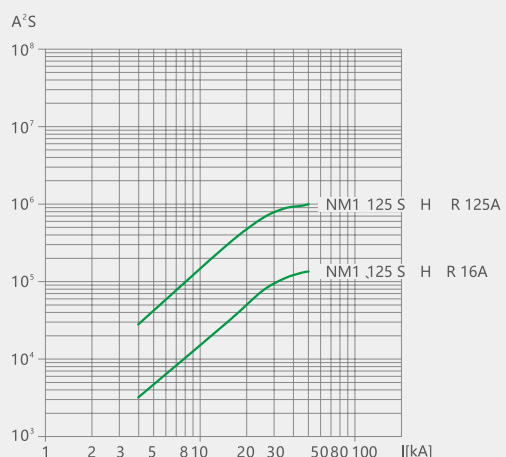
图 41 NM1-125 允通曲线
