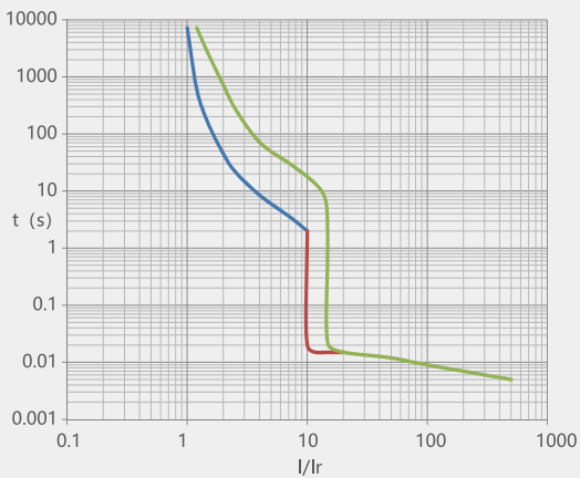
图 23 NM1-250 电动机保护
