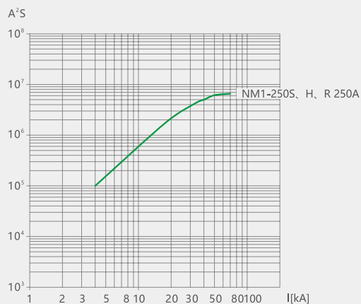
图 42 NM1-250 允通曲线
