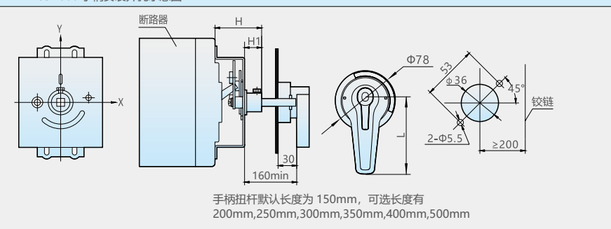
NM1-63~800 手柄安装开孔示意图
