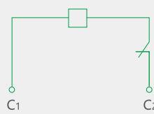
分励脱扣器接线图
