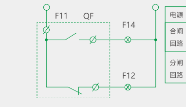
辅助触头接线图
