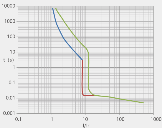
图 37 NM1-1250 配电保护
