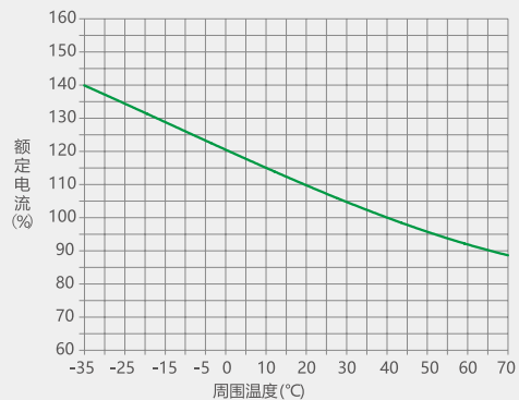
图 32 NM1-630 温度补偿曲线
