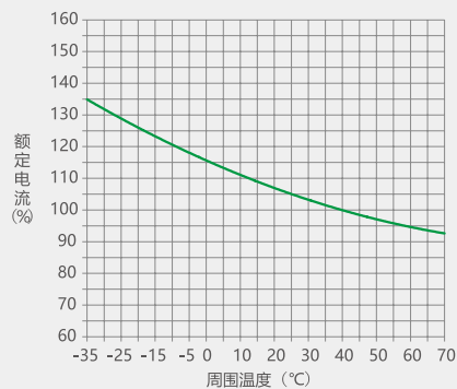
图 38 NM1-1250 温度补偿曲线
