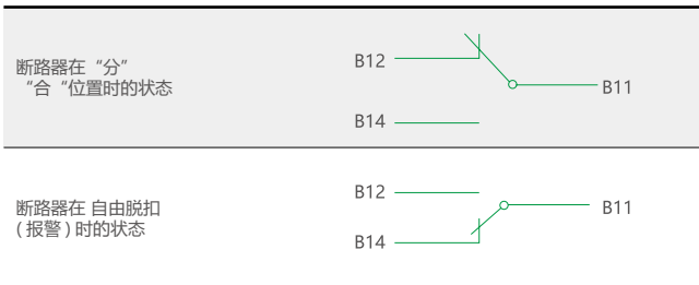
报警触头接线图
