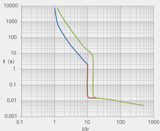
图 35 NM1-800 电动机保护
