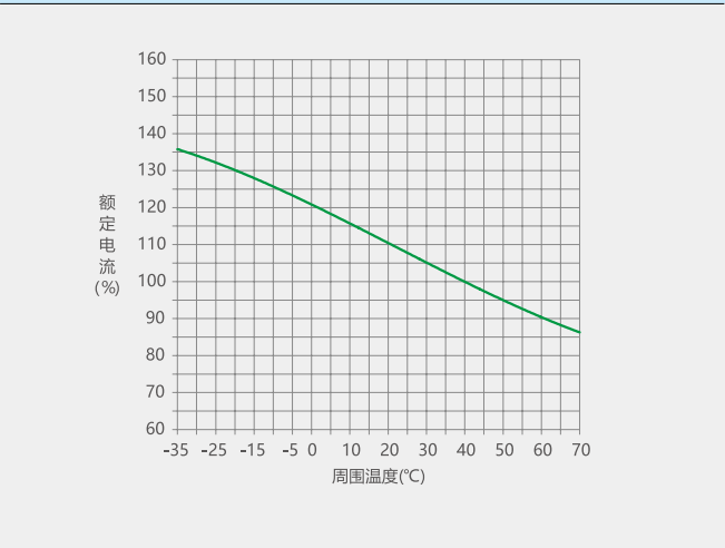
图 4 NM1-63 10A-25A 温度补偿曲线
