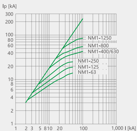
图 39 AC400V/415V 的 NM1 系列限流曲线图
