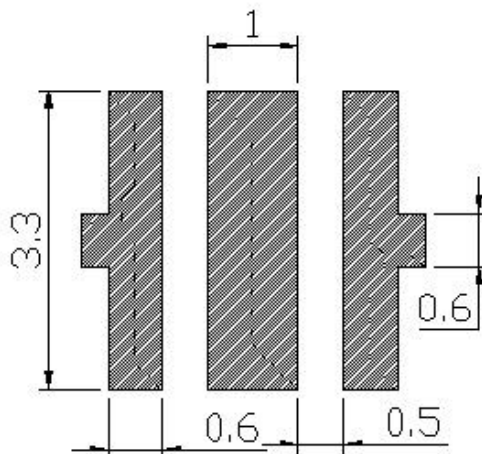
焊盘建议图
