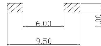
PCB. 焊接图
