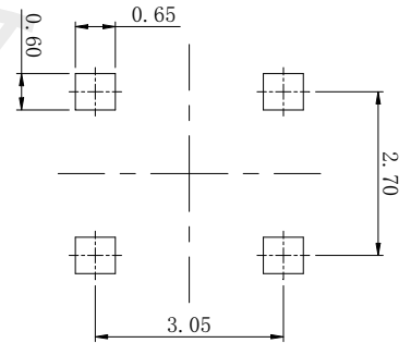
印刷板安装孔图 P.C.B Mounting pattern dimension
