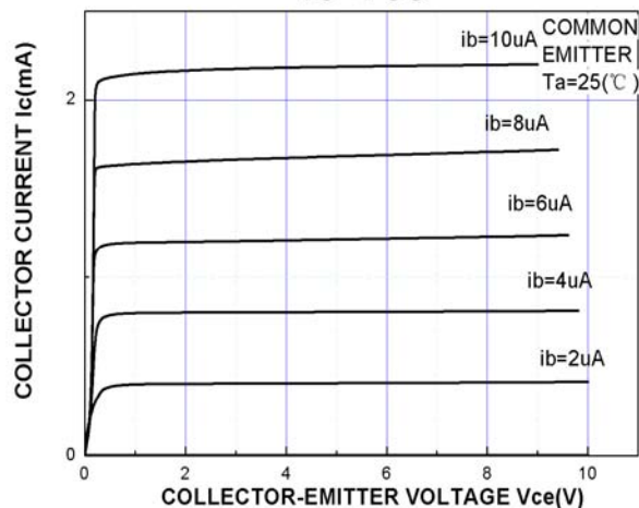
I c -V ce
