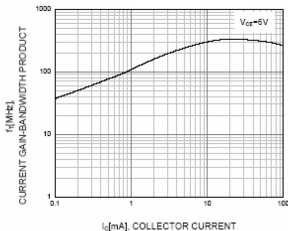
f T -I c
