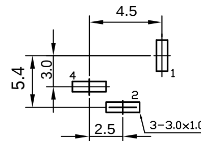
线路板安装尺寸示意图
