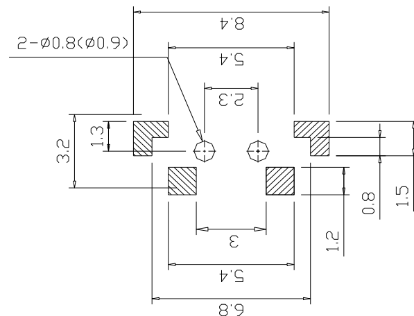
PCB. 焊接图
