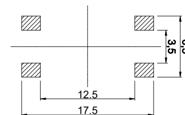
PCB. 焊接图
