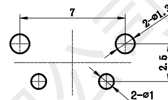
PCB线路板安装图(±0.1)
