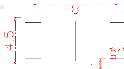
PCB. 焊接图
