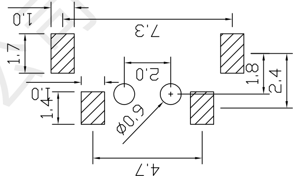
PCB. 焊接图
