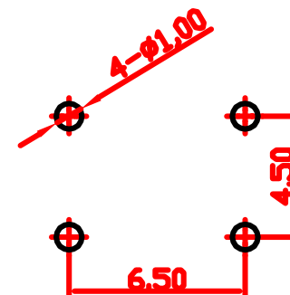
PCB. 焊接图
