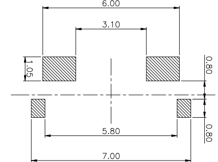
PCB. 焊接图
